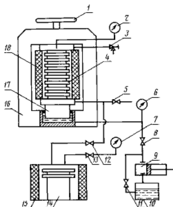
Схема автоклава типа АП-1
